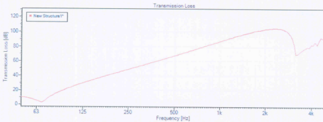
Рис.2 Частотная характеристика звукоизоляции конструкции №1
